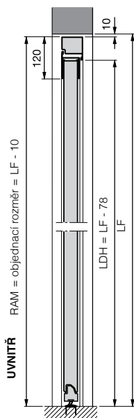
Ocelové vedlejší dveře Montáž za otvorem
