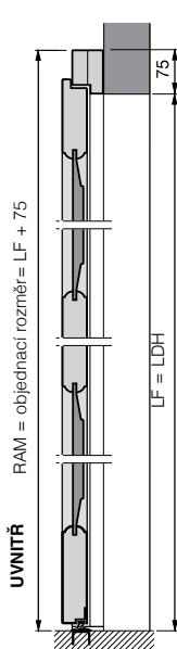
Dřevěné vedlejší dveře Montáž za otvorem
