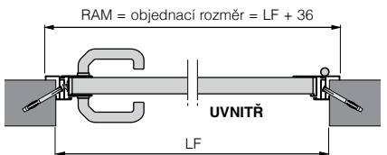
Ocelové vedlejší dveře s rohovou zárubeň Příklad vnějšího dorazu - typ profilu 3
