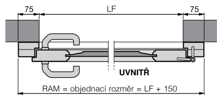
Dřevěné vedlejší dveře Montáž za otvorem
