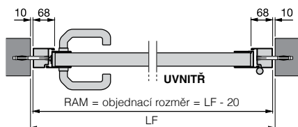
Ocelové vedlejší dveře Montáž v otvoru Příklad - typ profilu 2
