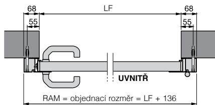
Ocelové vedlejší dveře Montáž v otvoru Příklad - typ profilu 2
